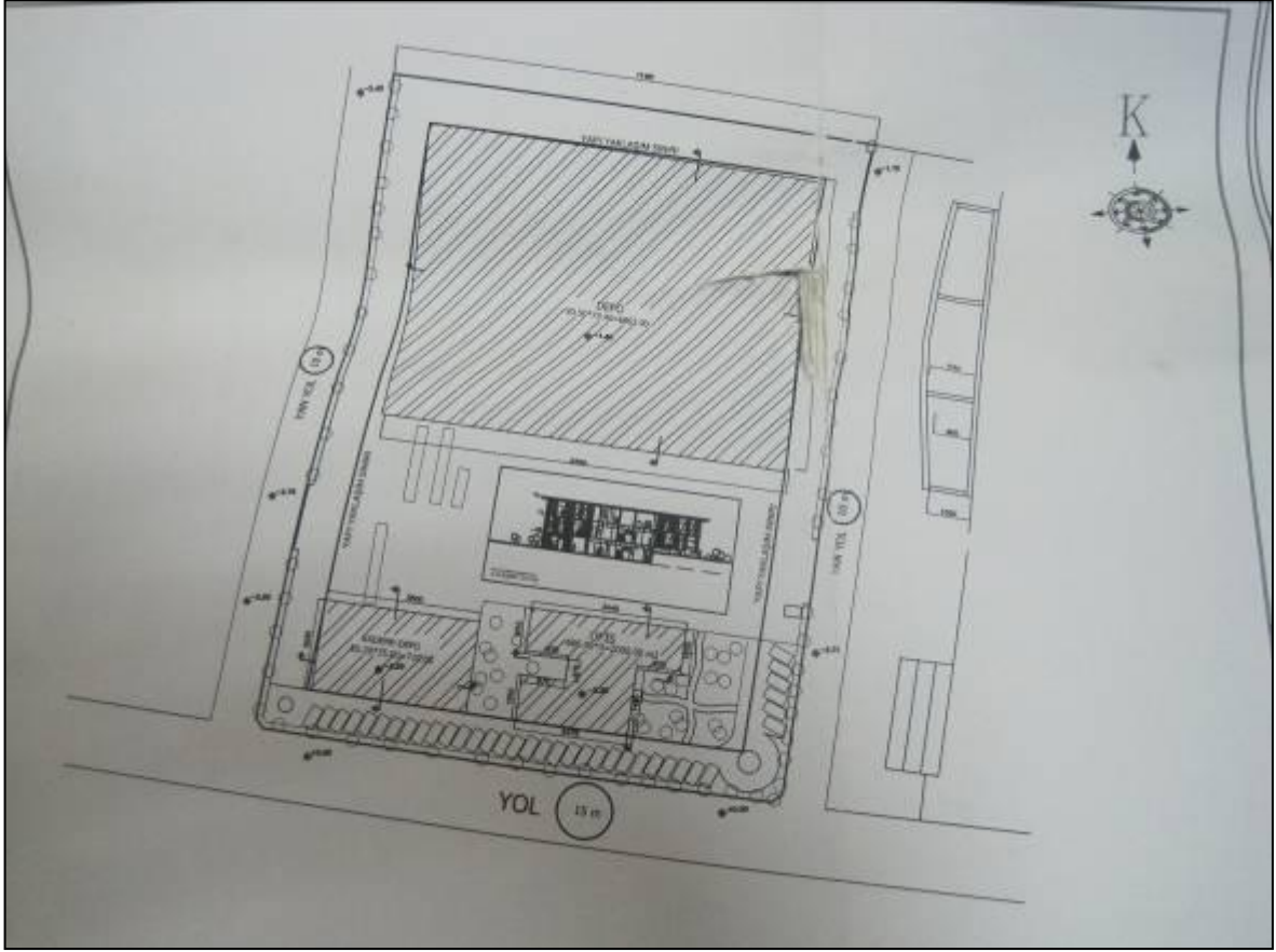
VAZİYET PLANI
