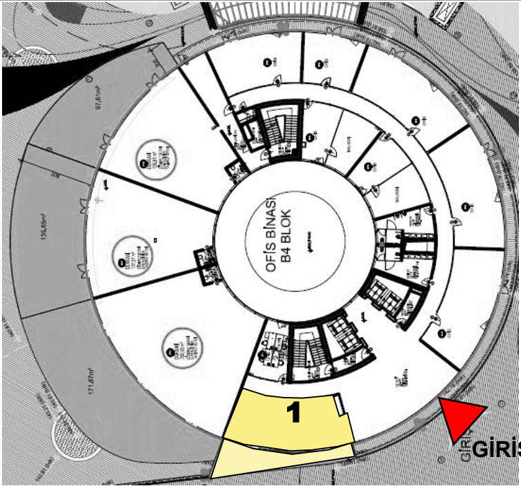
1. KAT PLANI
