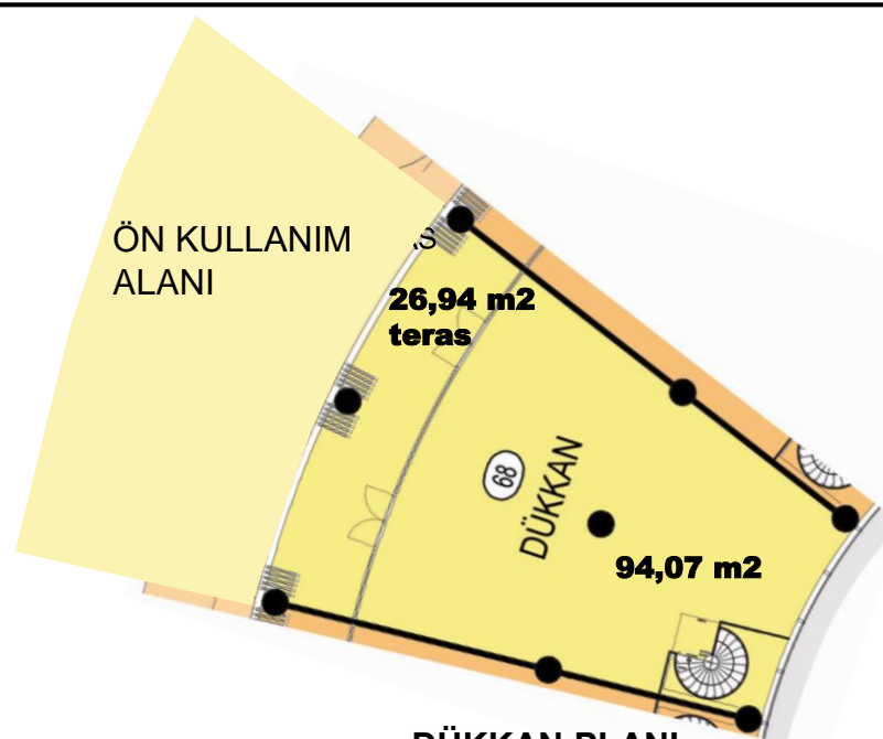
DÜKKAN PLANI
