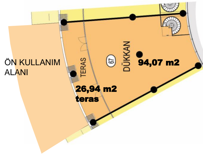
DÜKKAN PLANI
