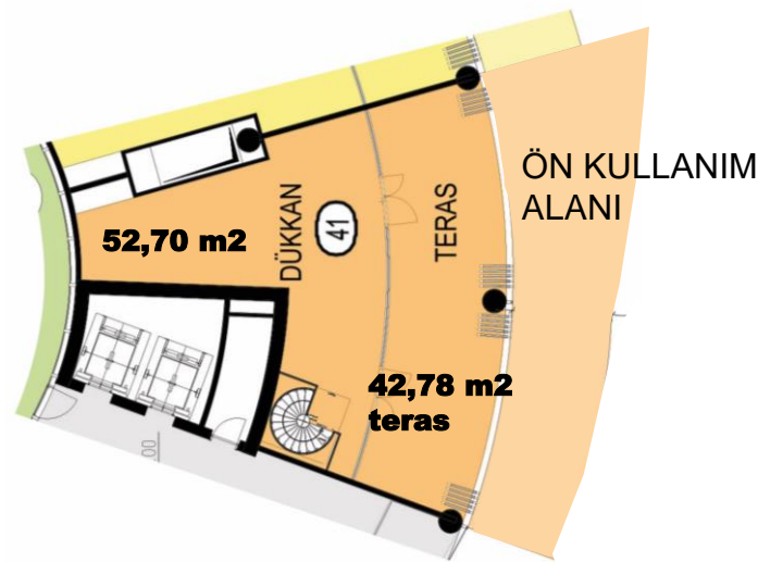
VAZİYET PLANI
