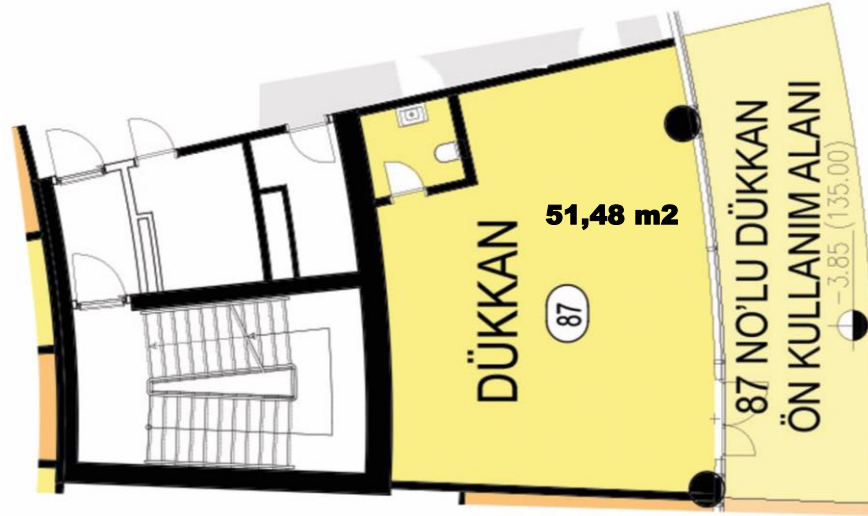
DÜKKAN PLANI
