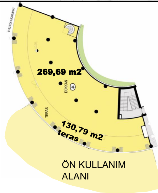
DÜKKAN PLANI
