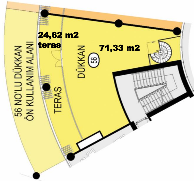
DÜKKAN PLANI
