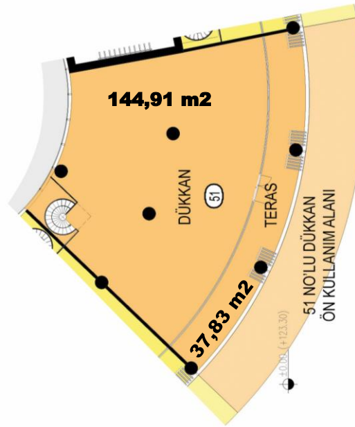
DÜKKAN PLANI
