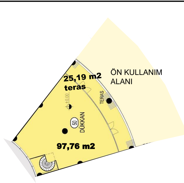
DÜKKAN PLANI
