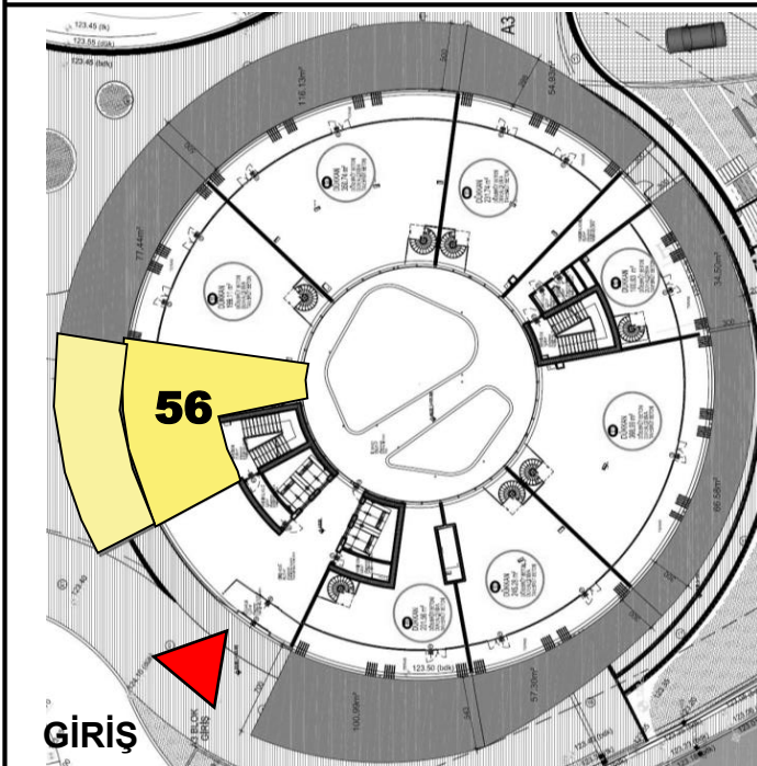
ZEMİN KAT PLANI
