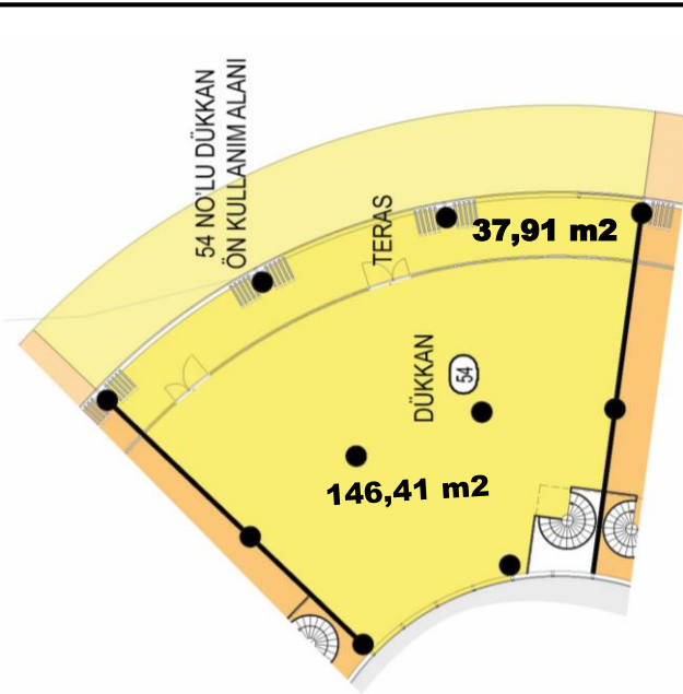
DÜKKAN PLANI
