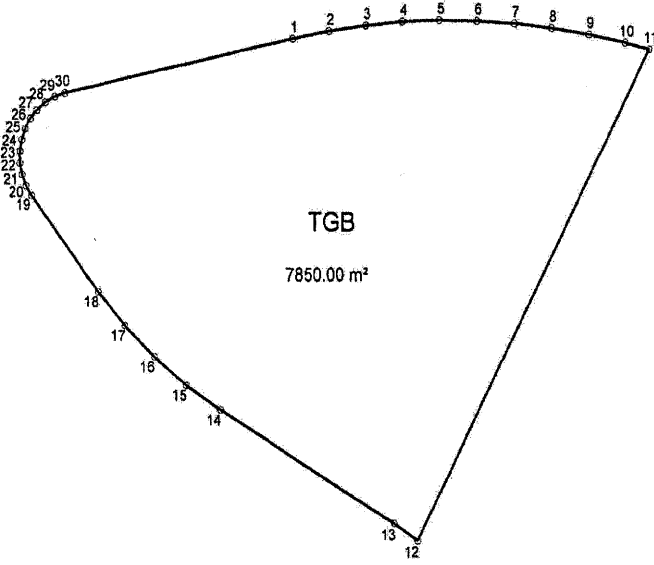
TGB ITRF KOORDİNAT ÖZETİ
